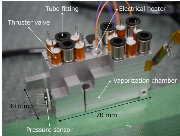
Figure 4. Vaporization chamber - EM
